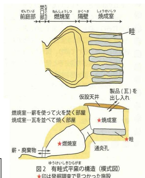
図 平窯の構造(『現地説明会資料』より) →
