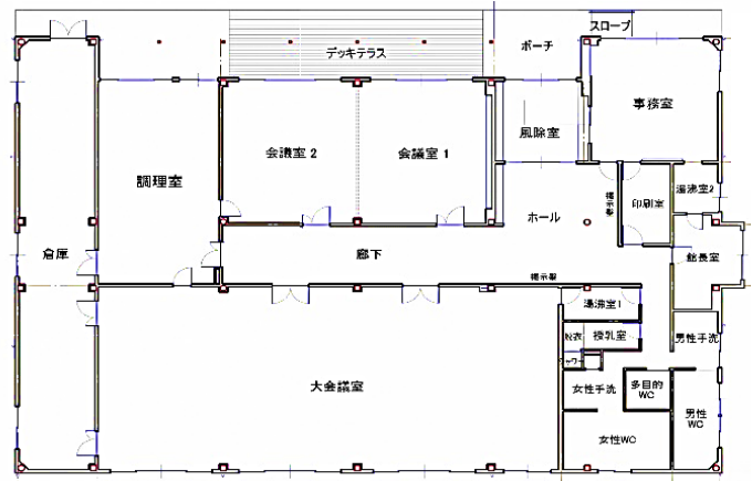
新竹矢公民館 平面図
