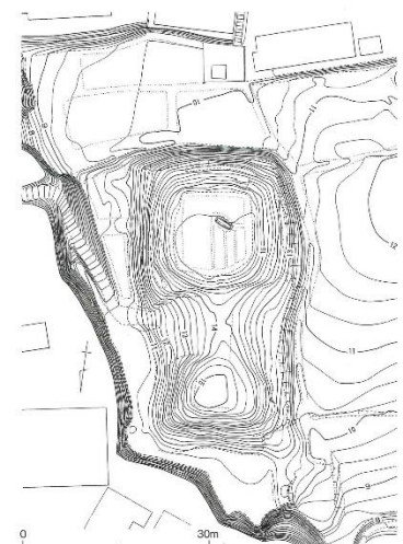
図2 測量図
