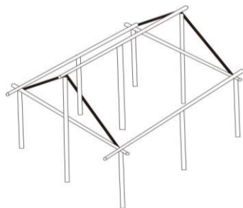
図 総柱建物の構造
