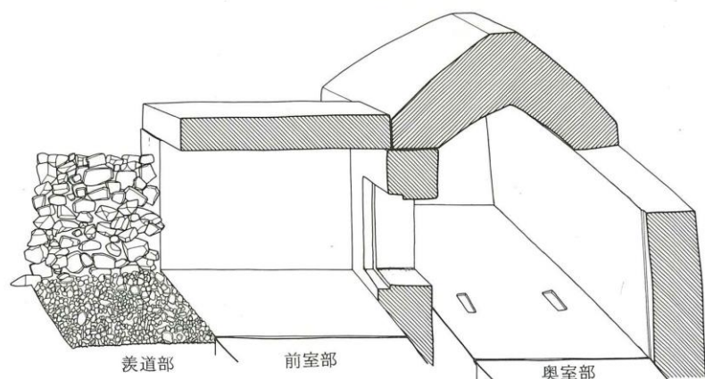
図：岩屋後古墳石室の復元図
