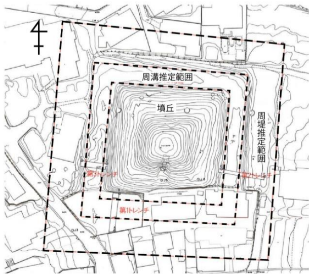
山代古墳の測量図
