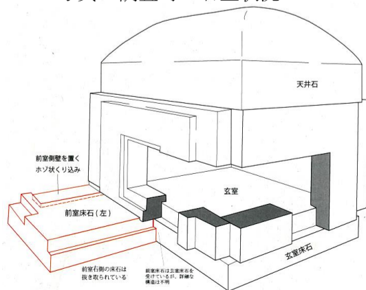
山代原古墳の石棺式石室模式図
