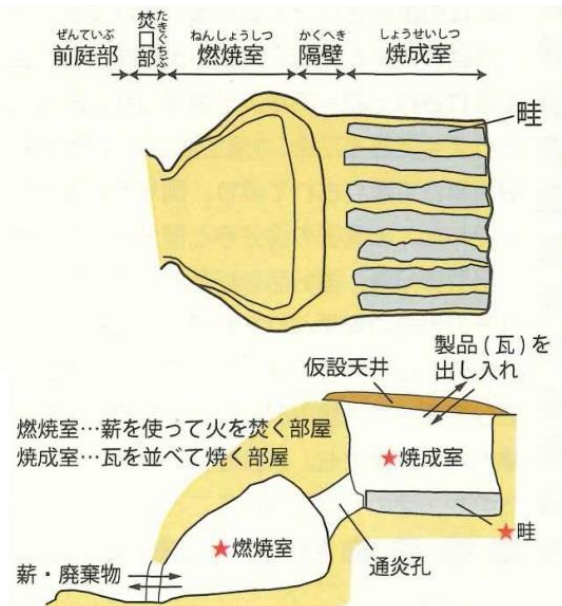
図2 有甕式平窯の構造(模式図)
