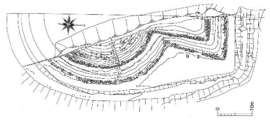
井ノ奥4号墳測量
